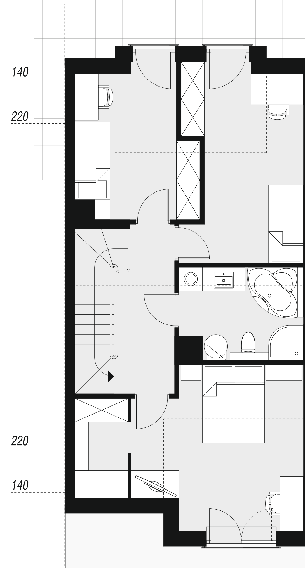
rzut poddasza
