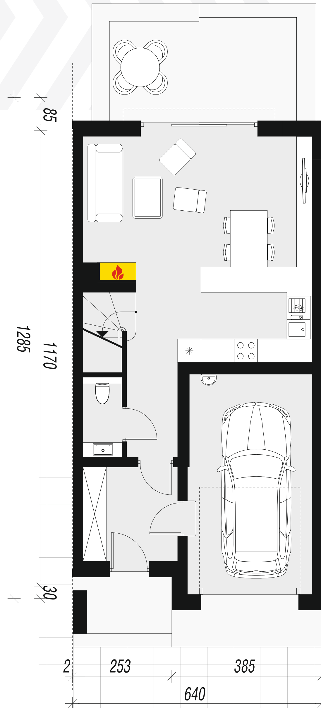
rzut parteru
